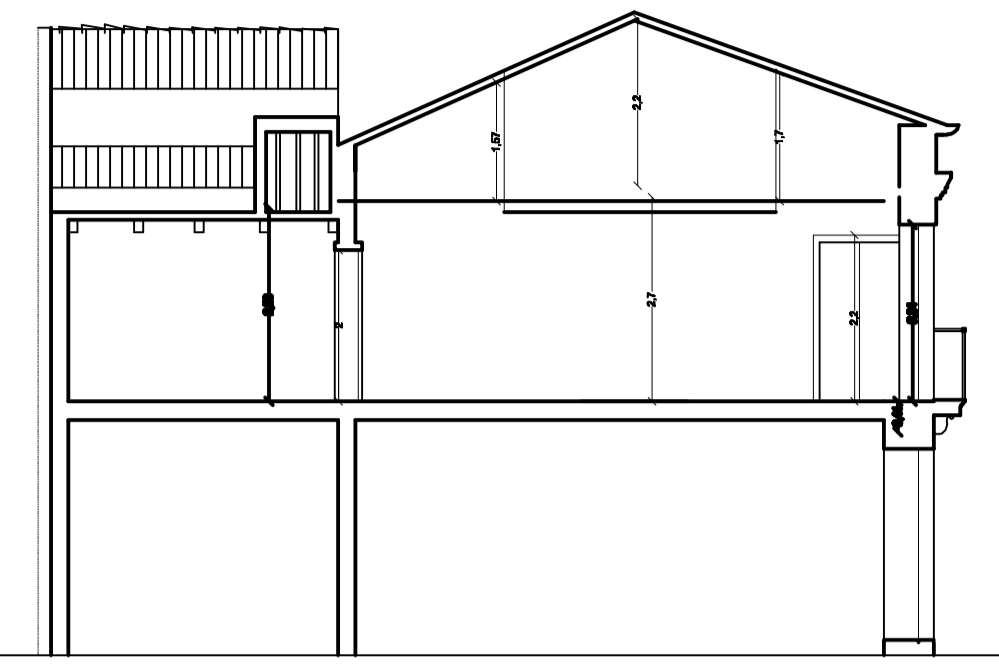
progetto sezione
