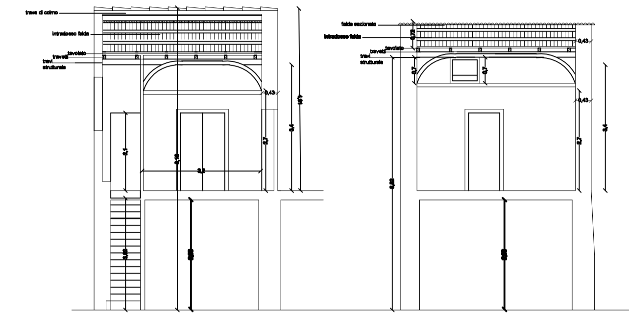
rilevo sezione
